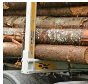
Enkel anpassning av vinkeln mellan banke och stötta maximerar lastförmågan vid transport av olika typer av last.
